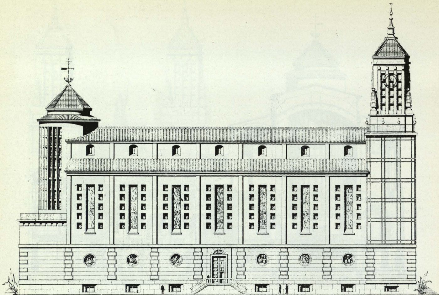
Fachada lateral.
