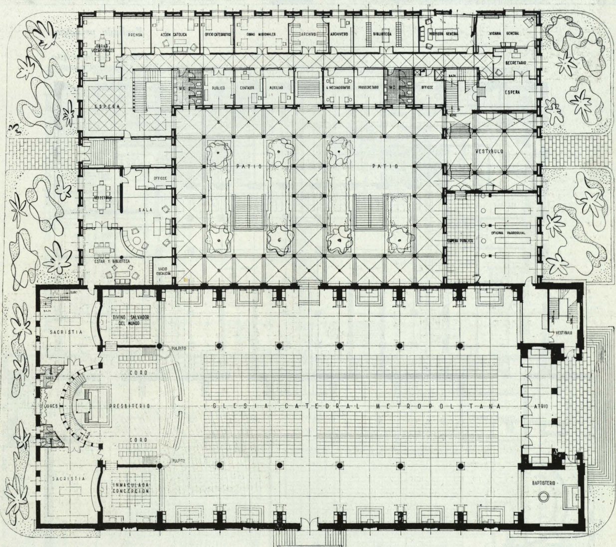
Planta baja.
