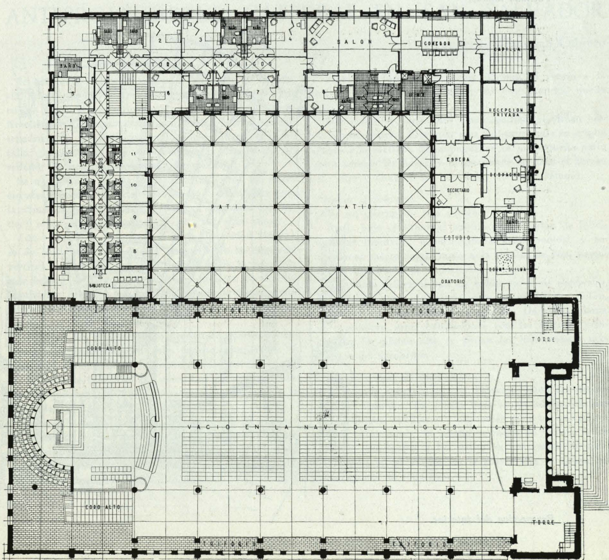
Planta alta.
