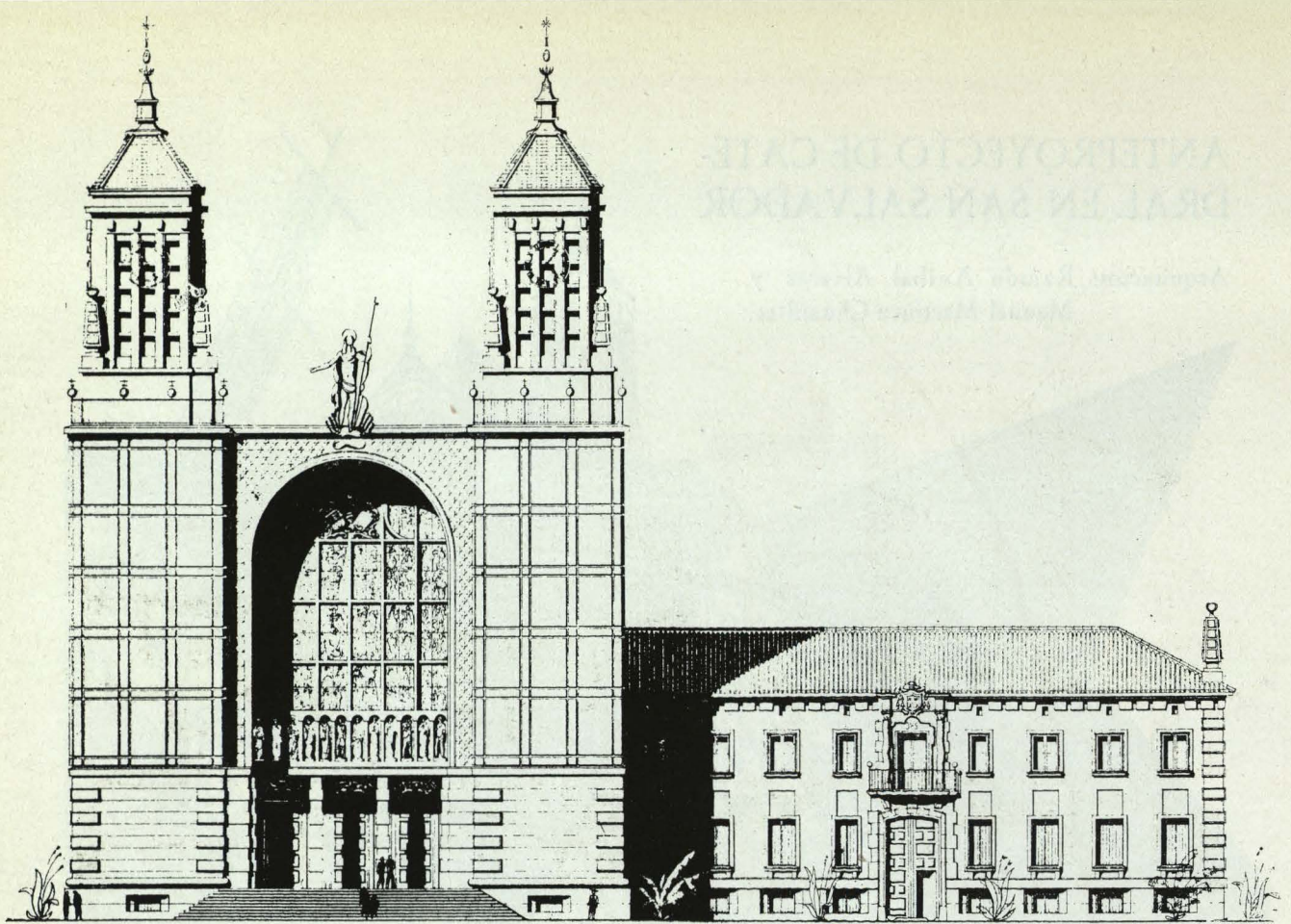
Fachada principal.
