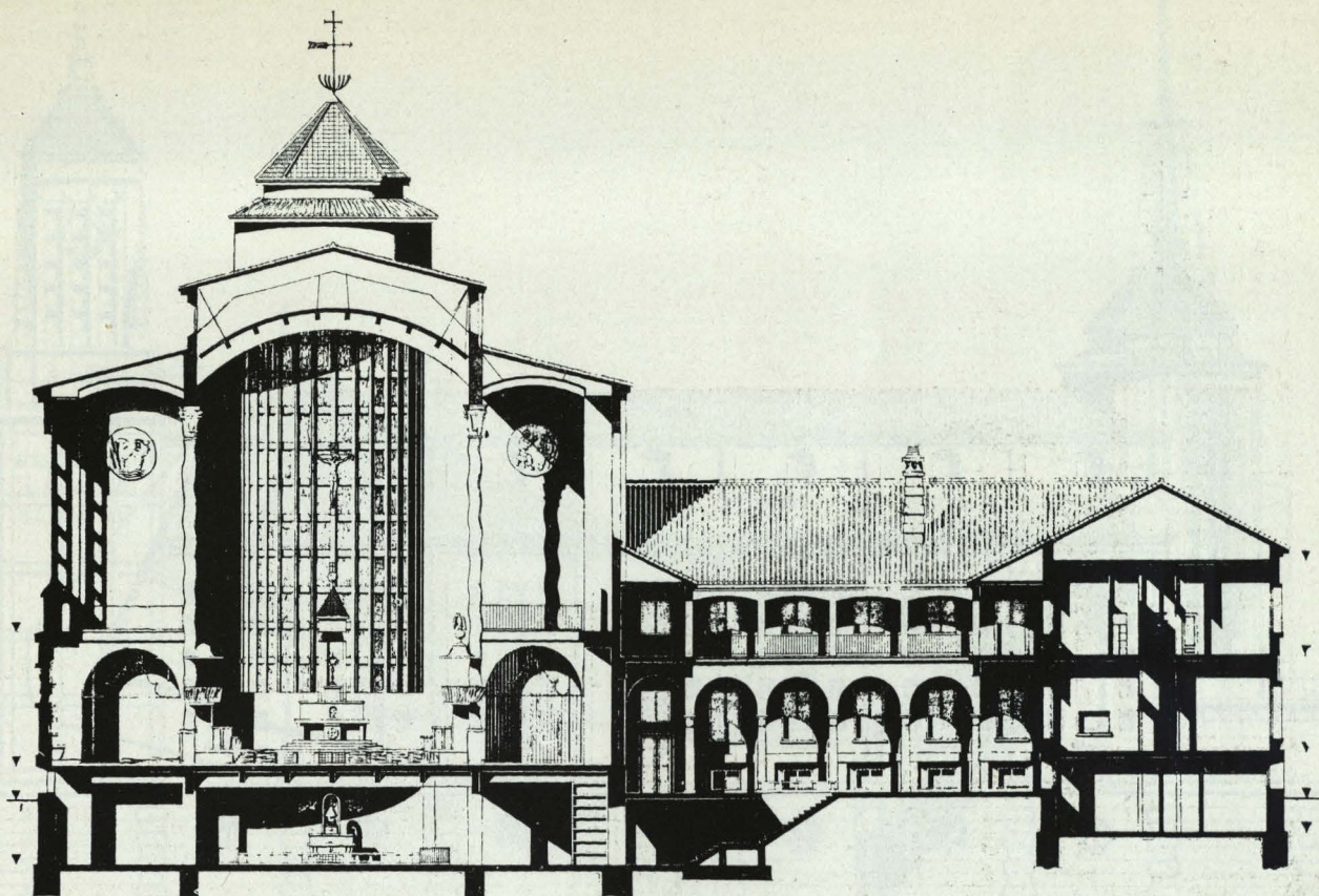
Sección longitudinal.
