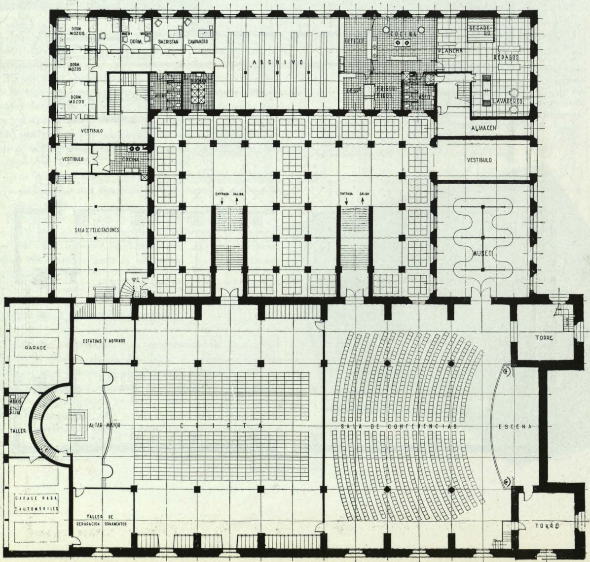
Planta de la cripta.
